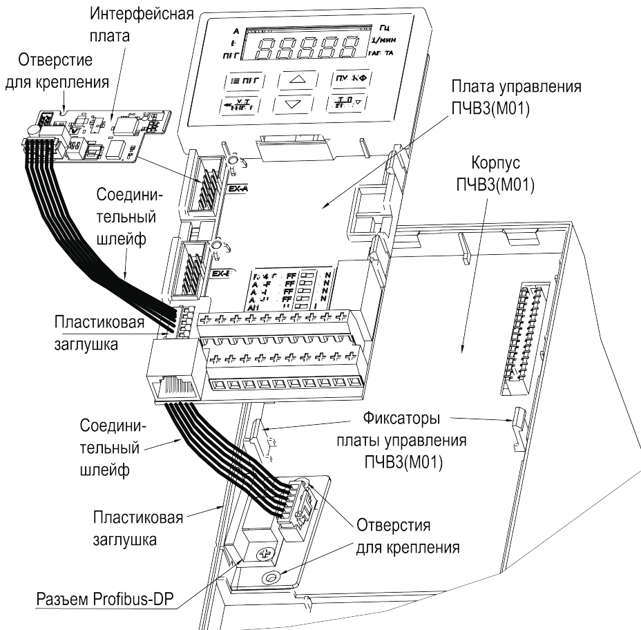
Рисунок 7.17 – Монтаж платы на преобразователях частоты мощностью до 45 кВт
