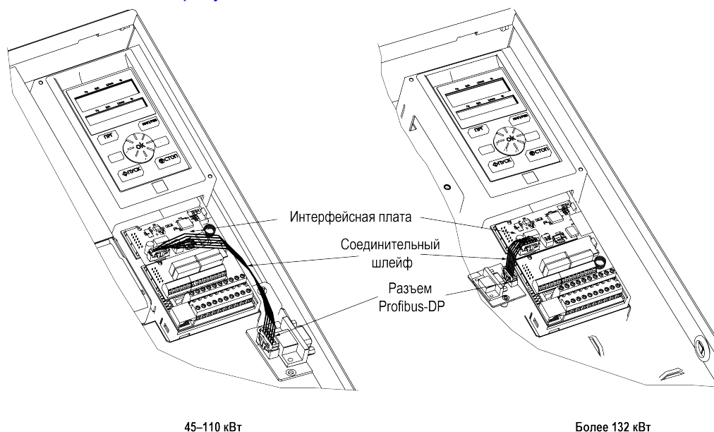
Рисунок 7.18 – Монтаж платы на преобразователях частоты мощностью более 45 кВт
