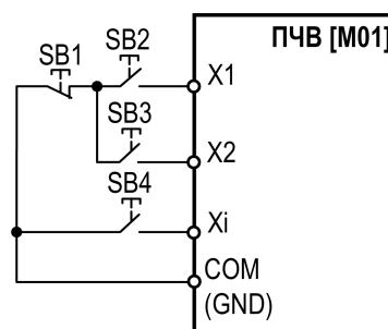
Рисунок 8.8 – Трехпроводная схема управления 1 (F05.20 = 2)
