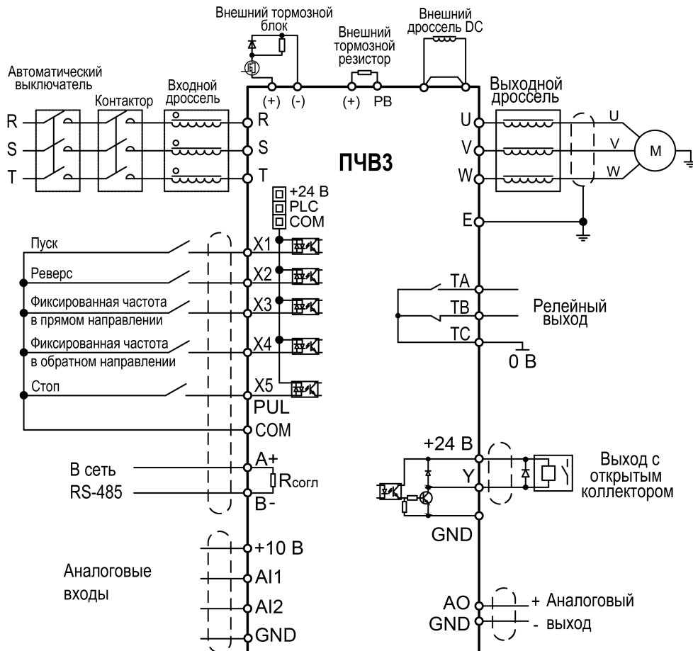
Рисунок 8.6 – Общая схема подключения
